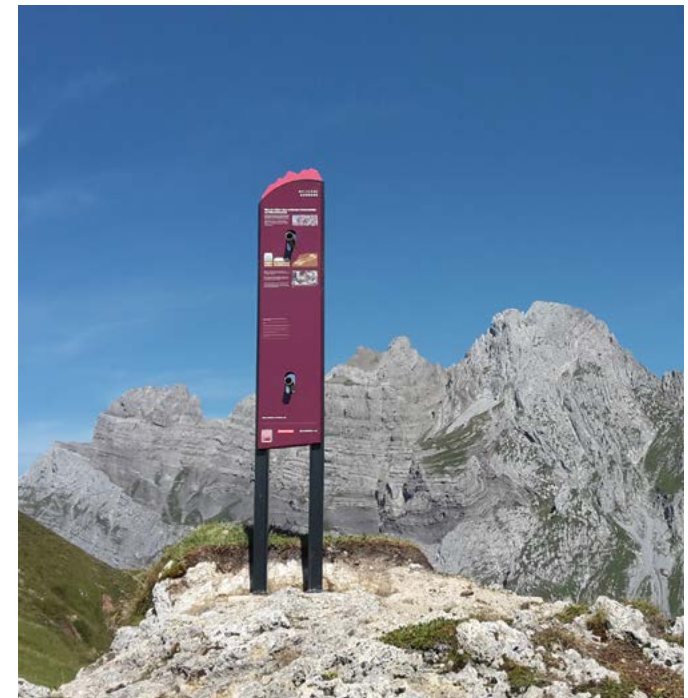
Sieben ausführliche Informationstafeln entlang der Wanderung erklären auf eindrückliche Weise und leicht verständlich die verschiedenen Geo-Phänomene.
